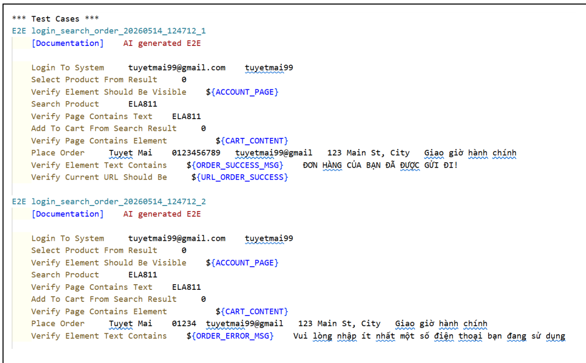
Hình 4.34 Test script chức năng Đặt hàng hoàn chỉnh
